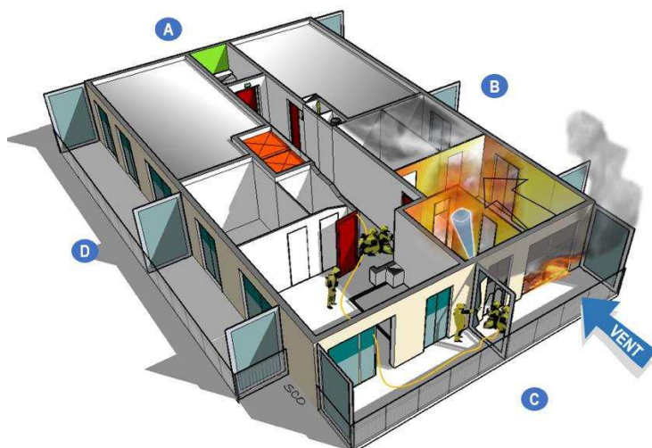
Schéma n°5 : feu démarrant sur un balcon avec rupture de la fenêtre et porte de l'appartement ouverte
